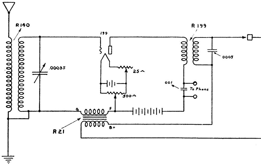
ALL-AMAX JUNIOR
